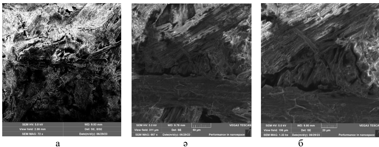
Сурет 18 - Бидай сабанынан волластонит қосылып жасалған қағаз үлгілерінің микрофотосуреттері
