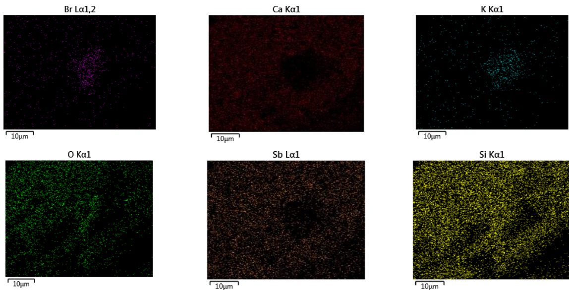
Сурет 21 – Волластониттің элементтік талдауының құрамы
