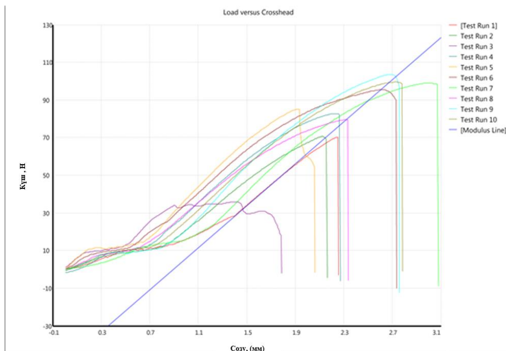
Сурет 45 - Үлгілердің созылу беріктігі
