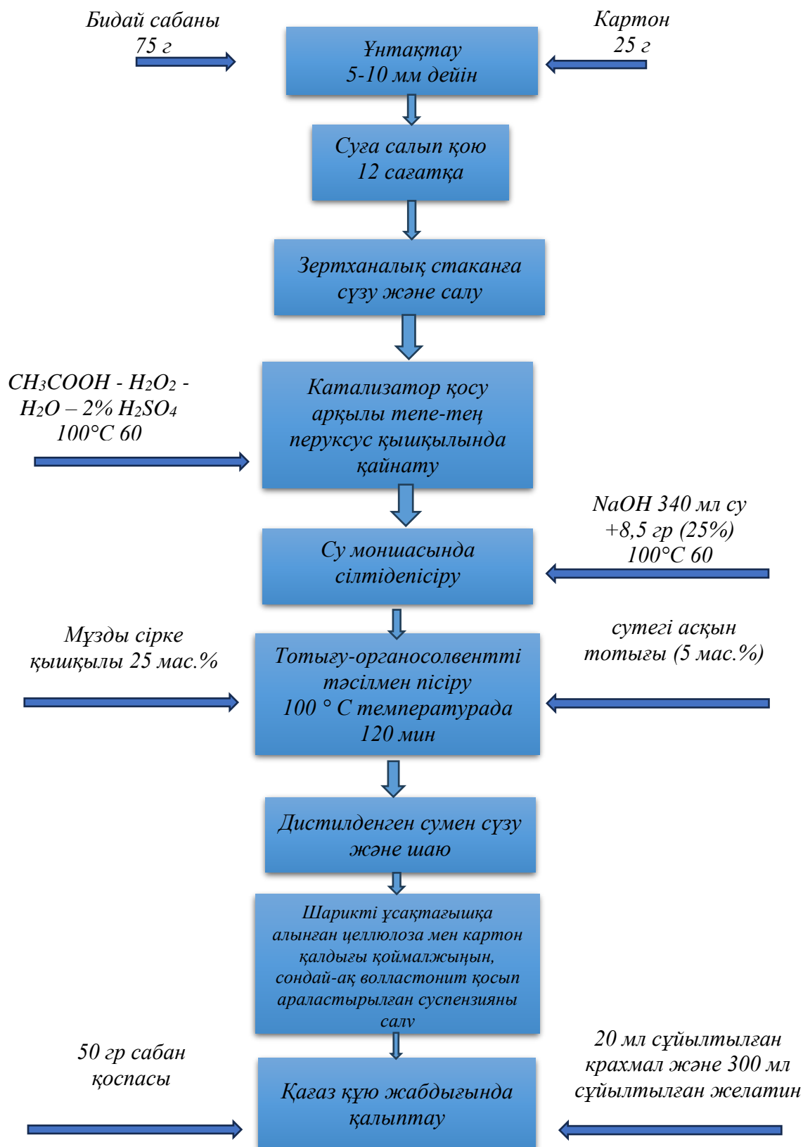
Сурет 22 - Бидай сабанынан картон мен волластонит қосылып қаптамаға арналған қағаз алудың технологиясы
