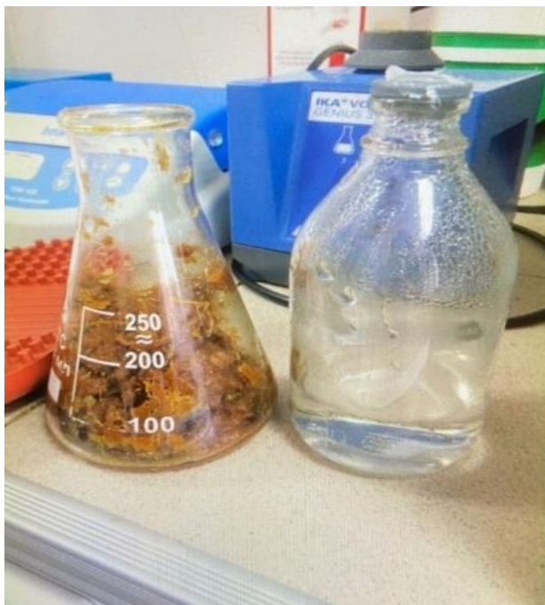
Сурет 27 - Тепе-тең перуксус қышқылының сулы ерітіндісі арқылы делигнификация
