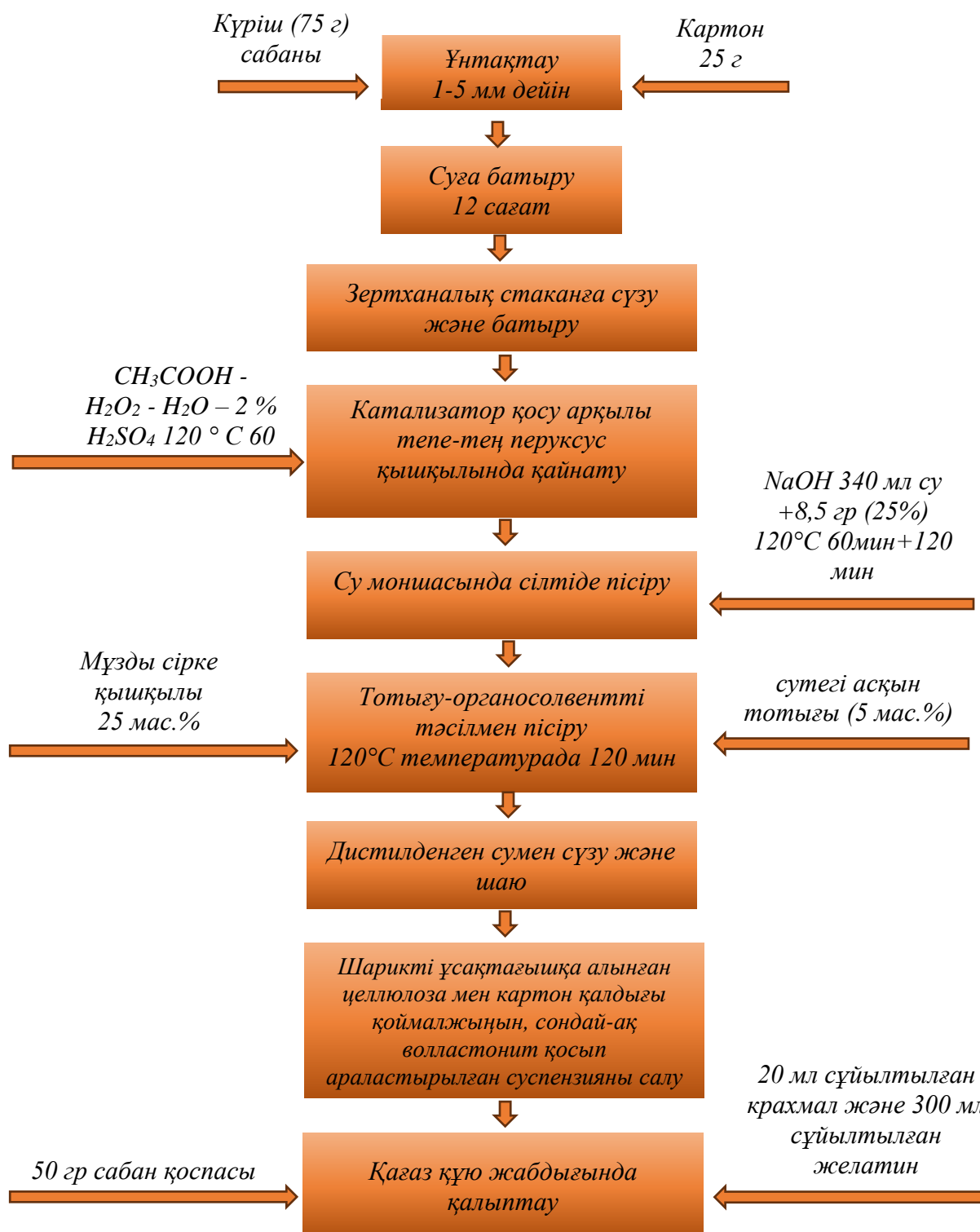
Сурет 25 – Күріш сабанынан картон мен волластонит қосылып қаптамаға арналған қағаз алудың технологиясы
