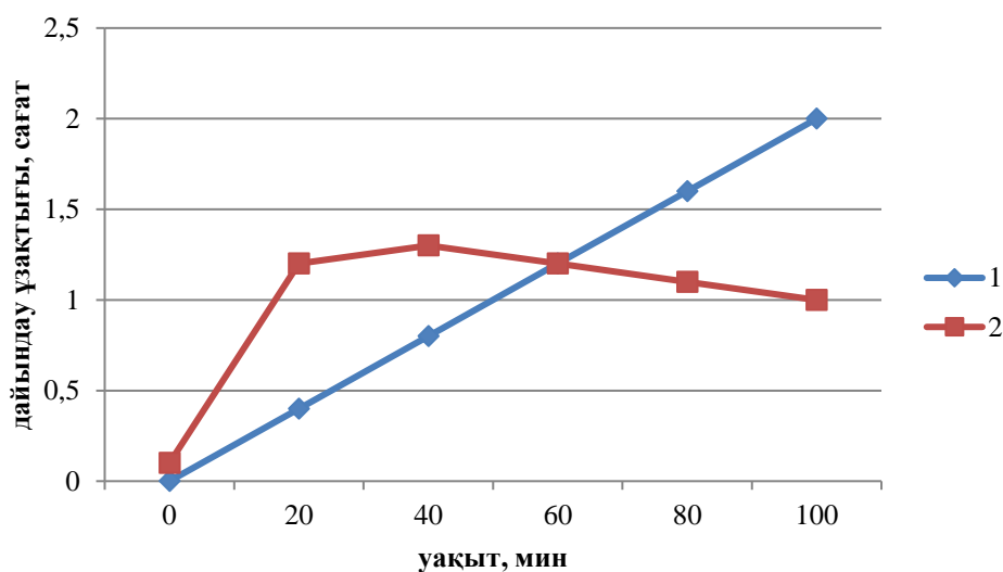
Сурет 34 – Тотығу-органосолвентті пісіру процесінің кинетикасын есептеу
