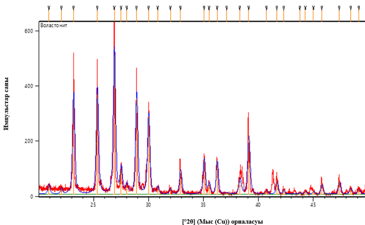
Сурет 20 – Волластонитті РФТ әдісімен талдау
