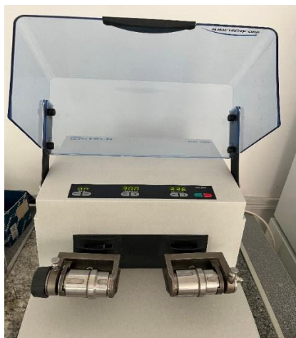
Сурет 10 - Шарикті диірмен
