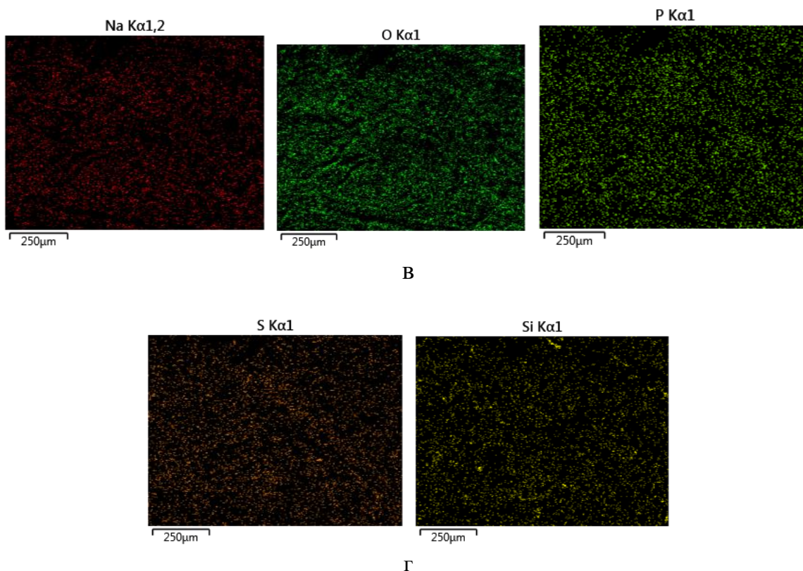
Сурет 36, парақ 2
