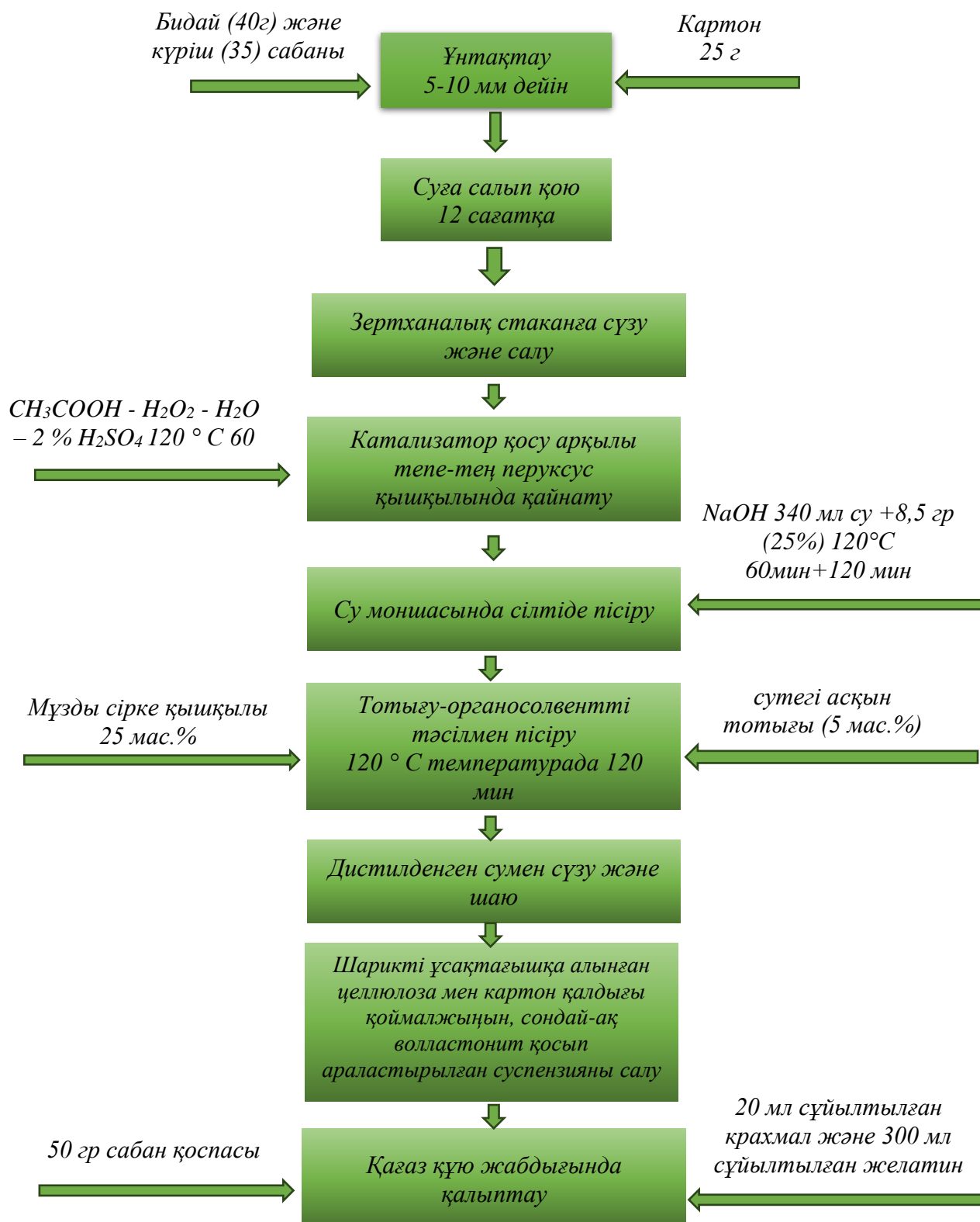
Сурет 24 – Бидай және күріш сабанынан картон мен волластонит қосылып қаптамаға арналған қағаз алудың технологиясы
