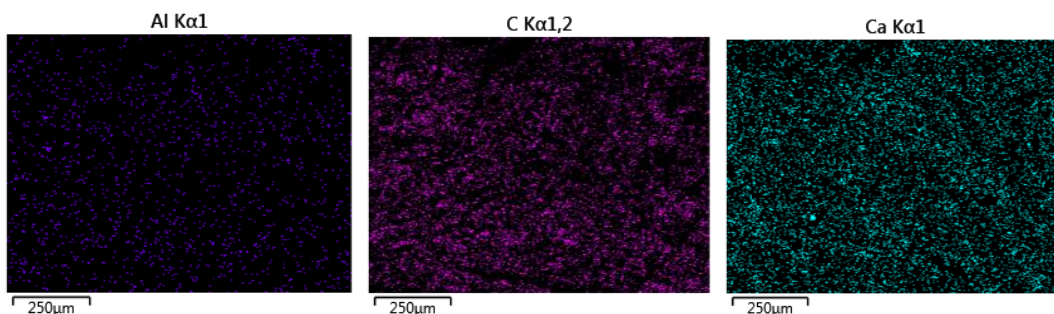
Сурет 36 - Бидай сабанынан жасалған қағаз үлгісінің элементтік құрамы, парақ 1
