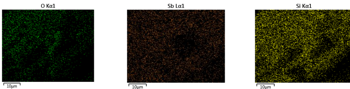
Сурет 21 – Волластониттің элементтік талдауының құрамы
