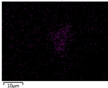
Br L \alpha 1,2
