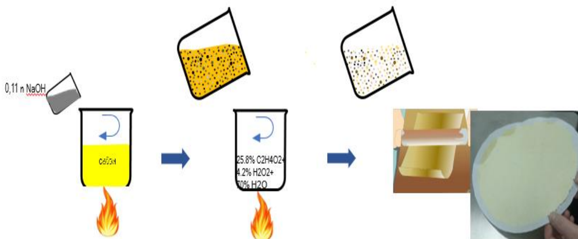
Сурет 26 - Зертханалық жағдайда сабаннан қағаз жасау процесі
